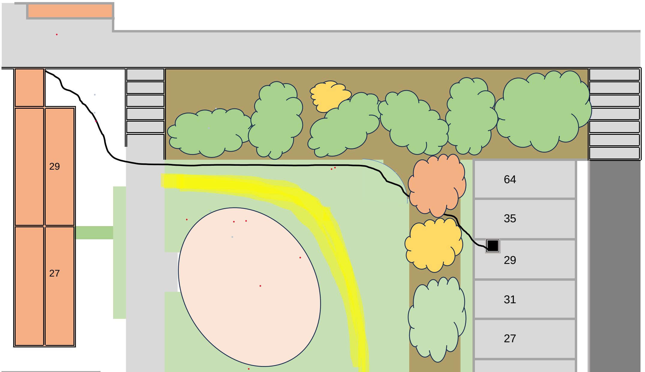
Kabelføring til Ladestander Vognly EKV 29
